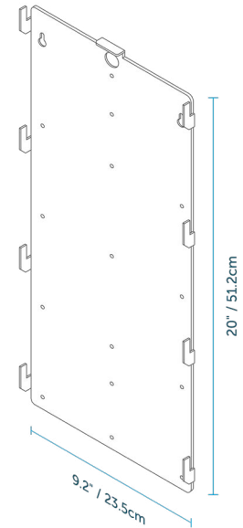
背面パネル
